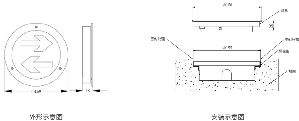
关键尺寸图 (mm)
