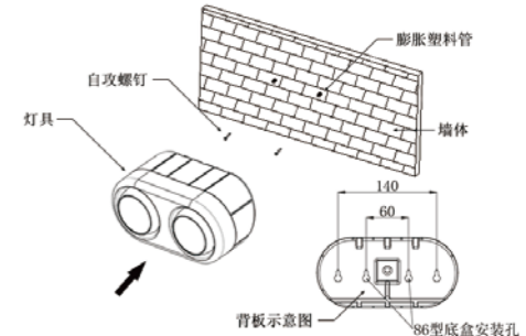
双头灯安装示意图
